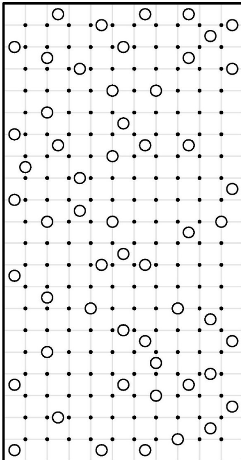
کهکشان ۱۰
