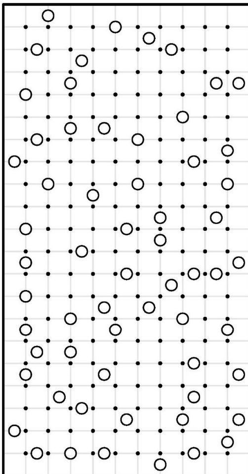
کهکشان ۲
