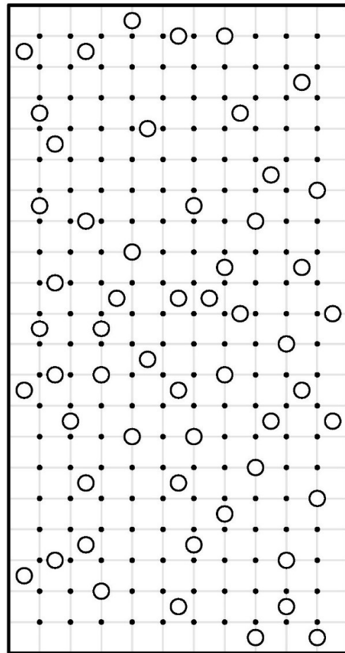
کهکشان ۳
