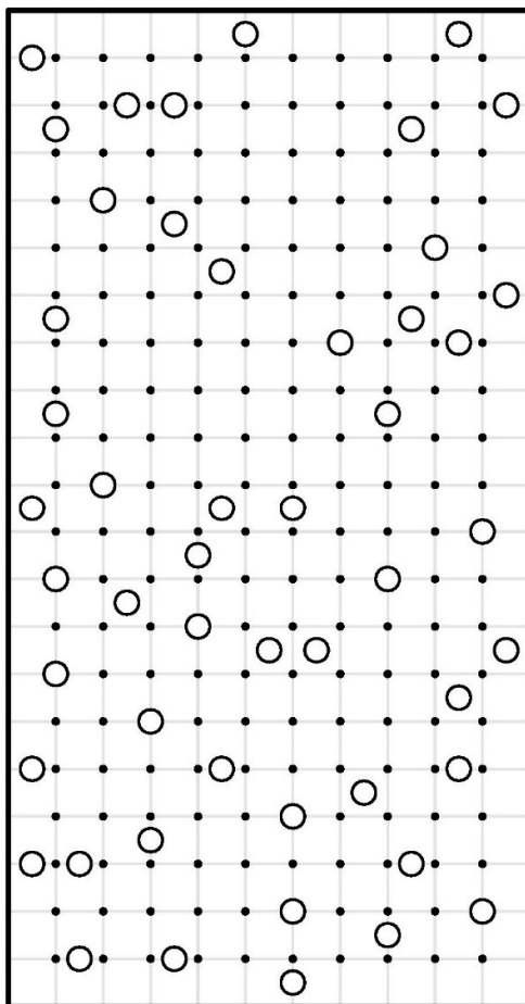
کهکشان ۶
