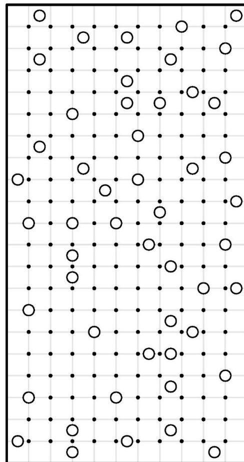
کهکشان ۵
