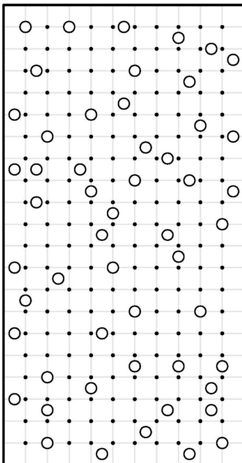
کهکشان ۱۲
