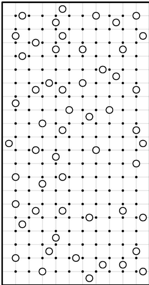
کهکشان ۴
