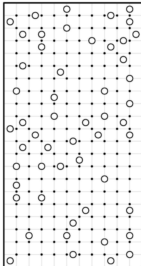
کهکشان ۱۱
