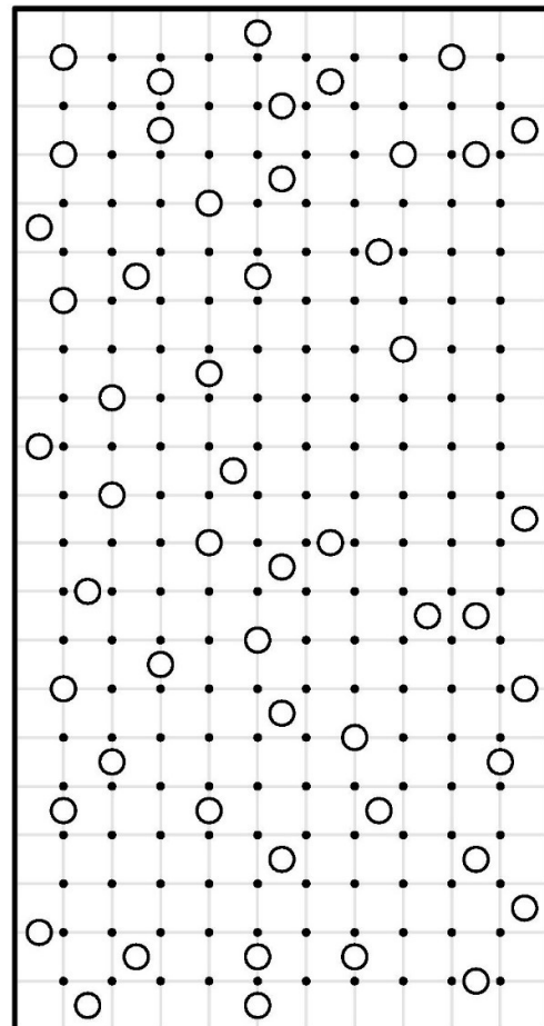
کهکشان ۷
