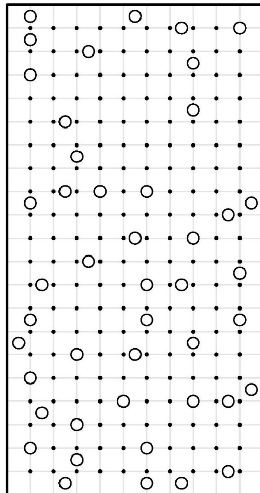
کهکشان ۱
