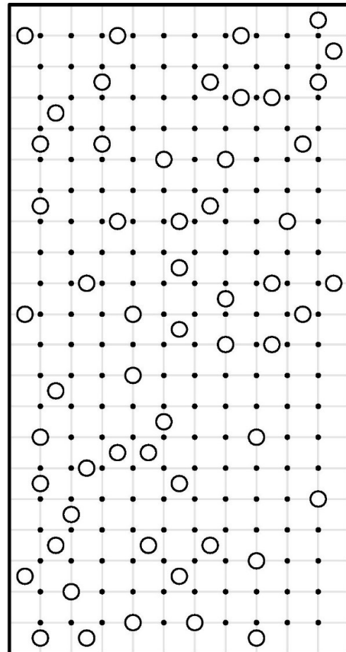
کهکشان ۹
