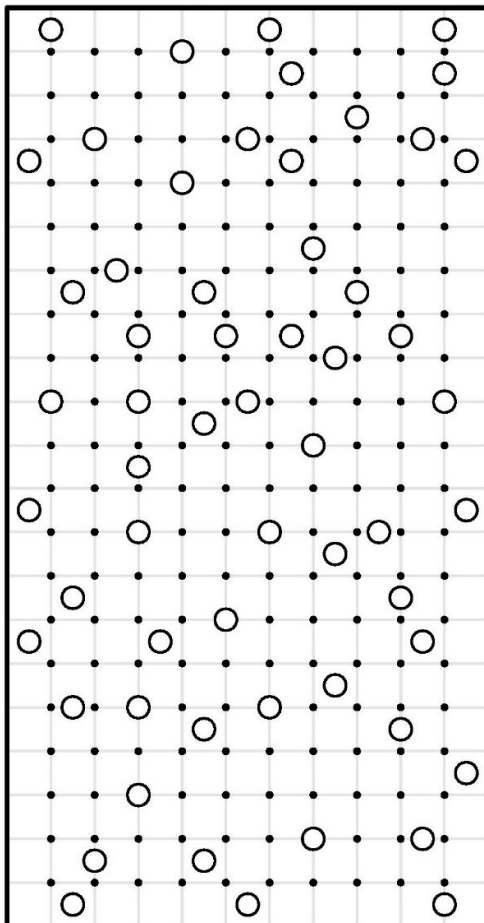
کهکشان ۸
