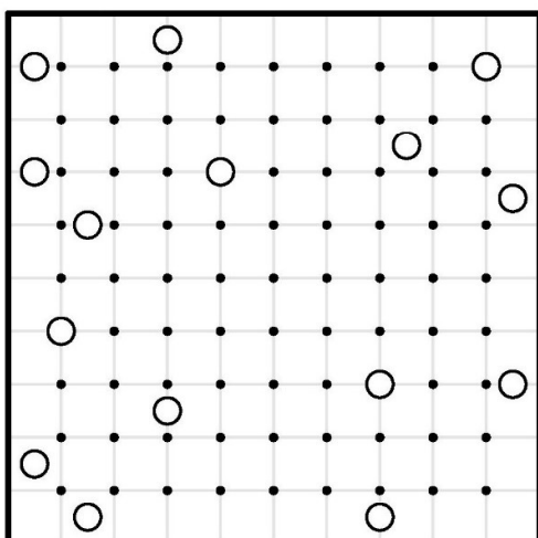
کهکشان ۴
