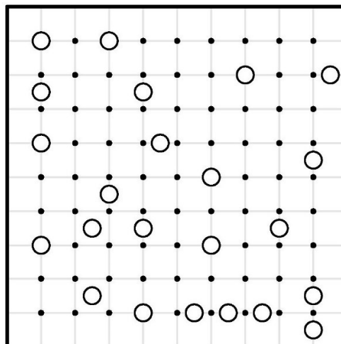
کهکشان ۵
