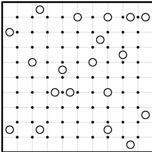
کهکشان ۱۰
