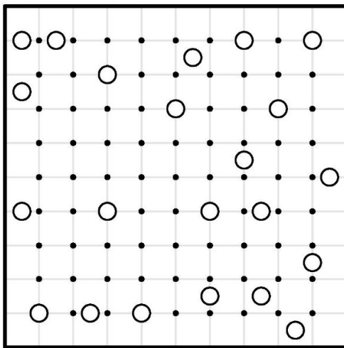
کهکشان ۱۴
