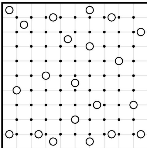
کهکشان ۱۶
