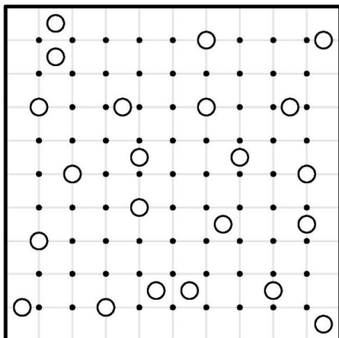
کهکشان ۶
