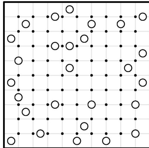
کهکشان ۹
