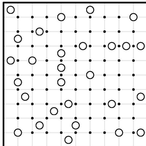
کهکشان ۱
