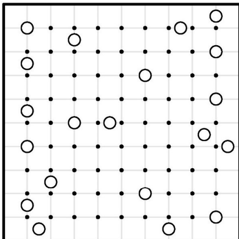
کهکشان ۲
