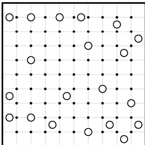
کهکشان ۸
