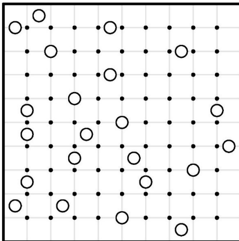
کهکشان ۱۲
