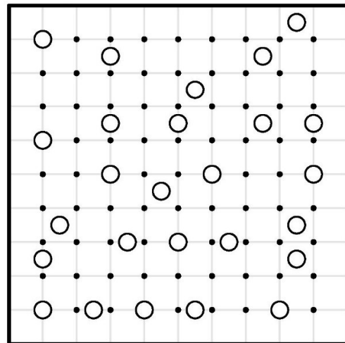
کهکشان ۱۱
