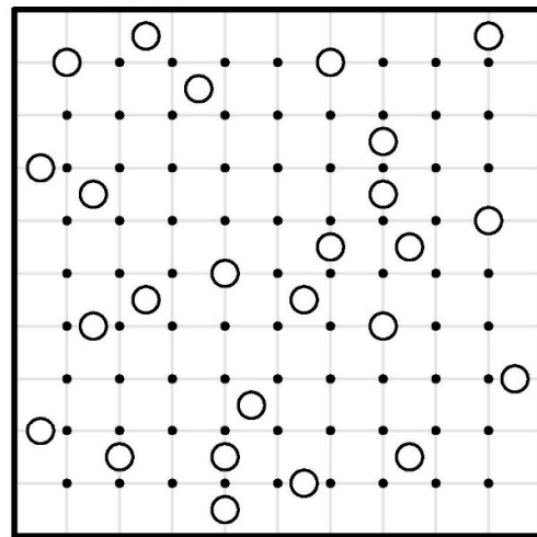
کهکشان ۱۳
